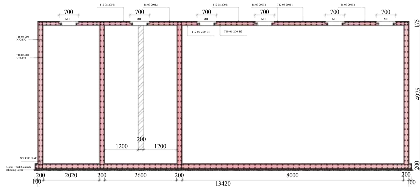
SECTION A-A
