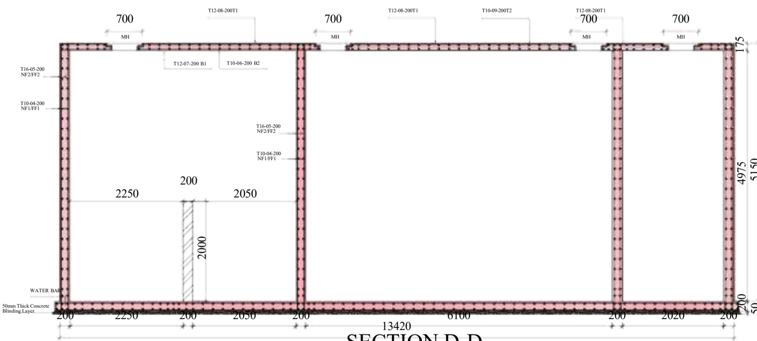
SECTION D-D
